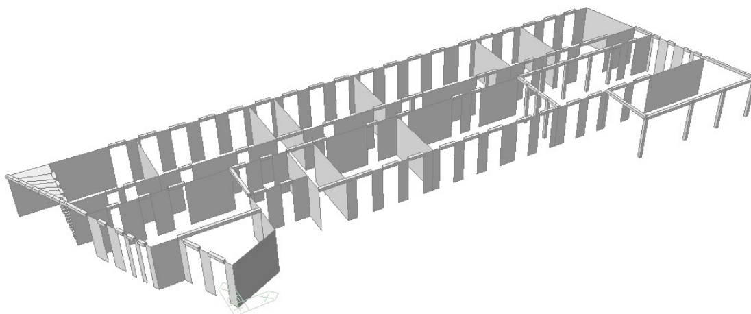
Figura 7 – Vista del modello FEM del Corpo Uffici
