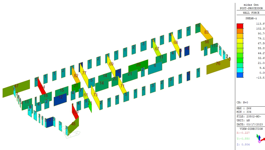
Figura 14 - Taglio sollecitante Fz – Involuppo Comb. Sismiche Y
