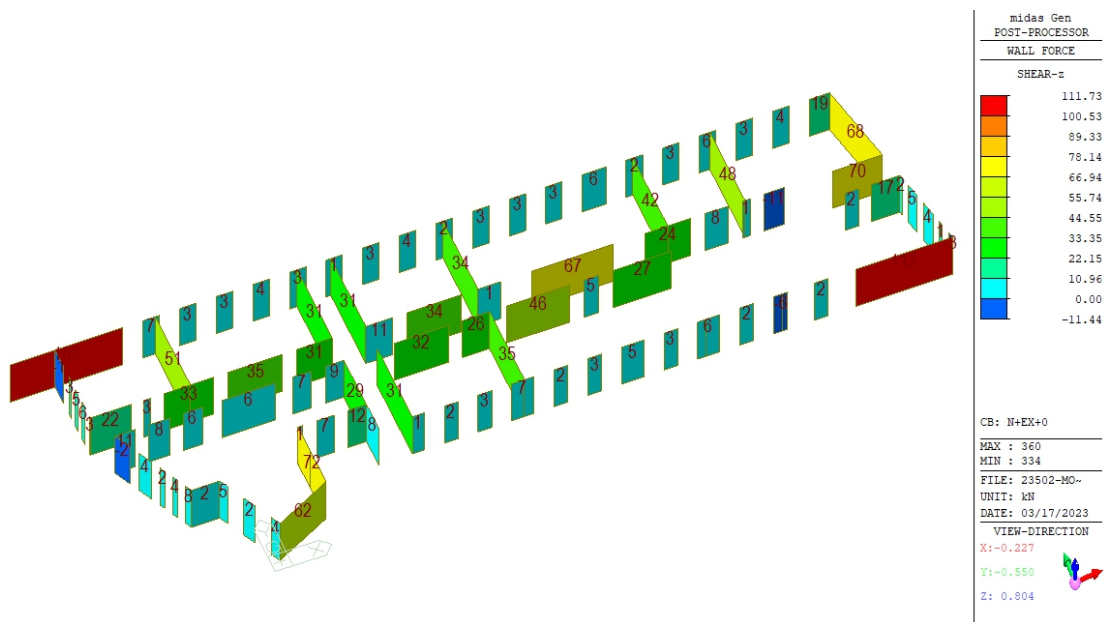
Figura 13 – Taglio sollecitante Fz – Involuppo Comb. Sismiche X
